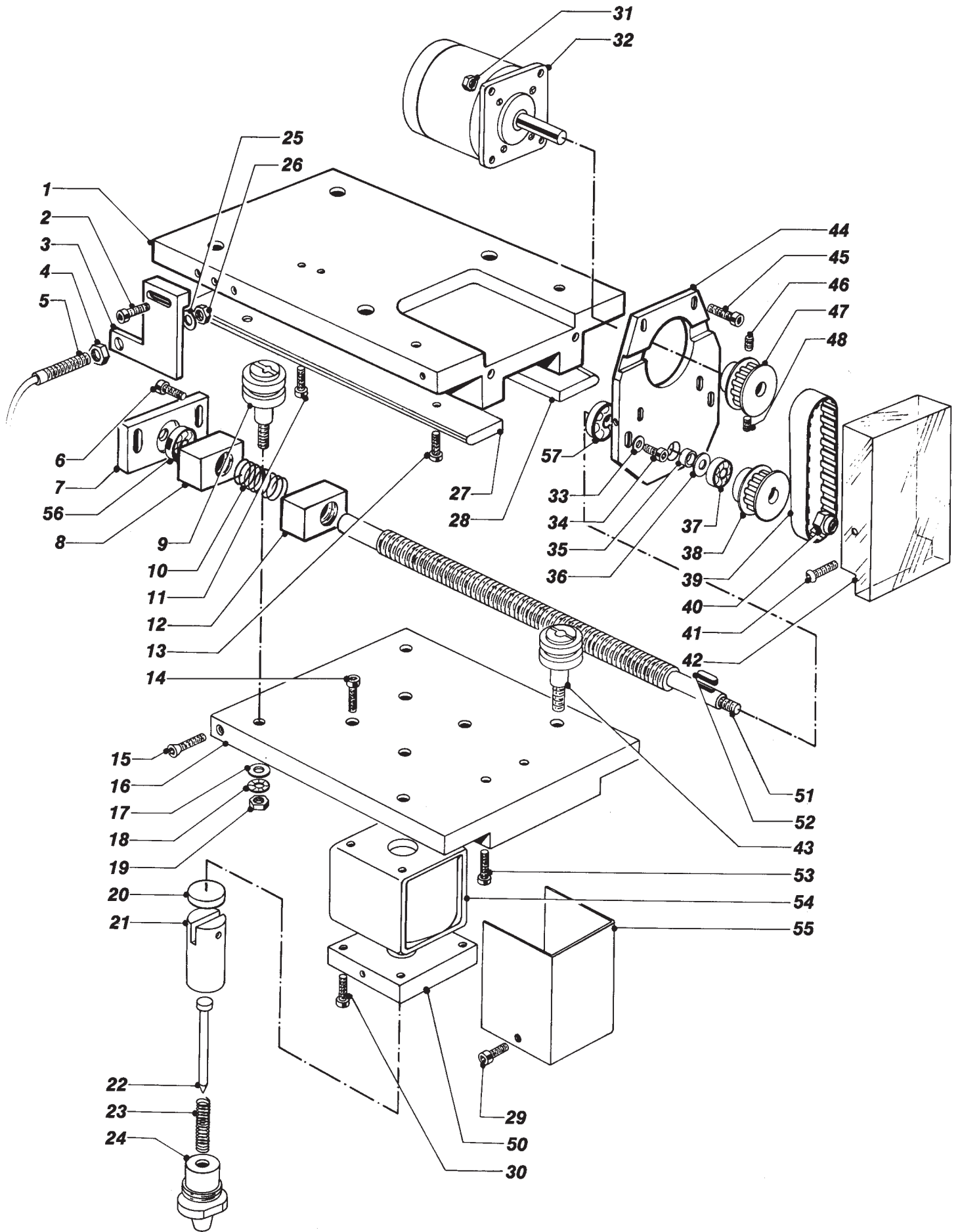
Disegno pubblicato per gentile concessione della Società SOMAUT - Macchine per Marcare
