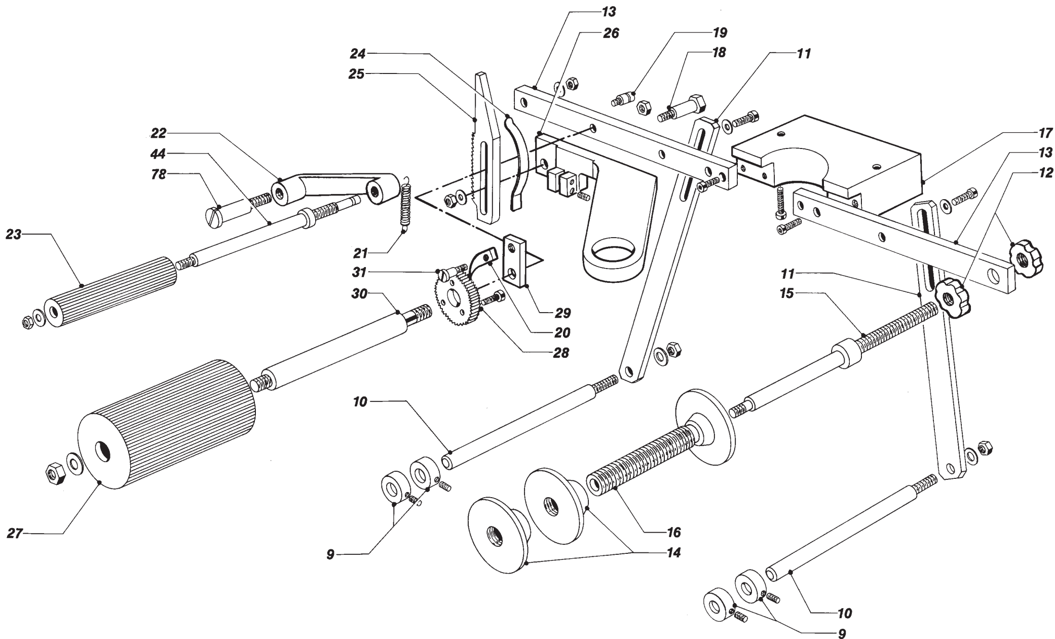
Disegno pubblicato per gentile concessione della Società SOMAUT - Macchine per Marcare
